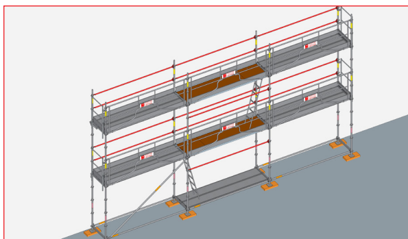
Montage Lisse KLMR sur gamme MULTISECU+
