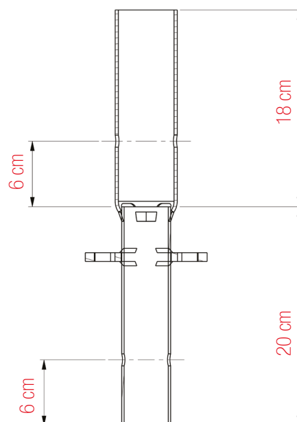
COUPE A-A
