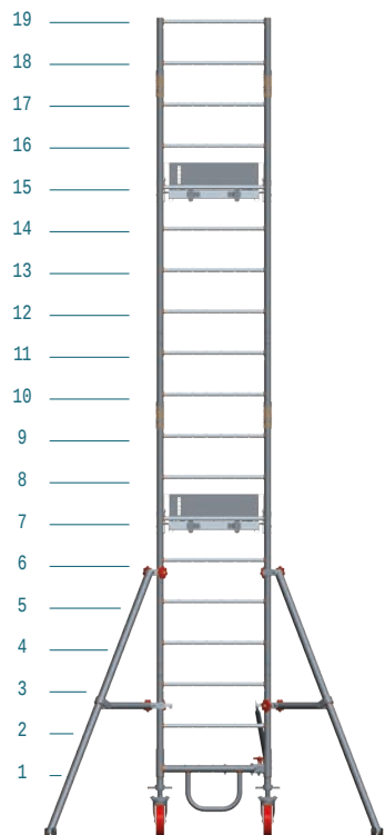
- Position d'accrochage des stabilisateurs (R SECU 200)
