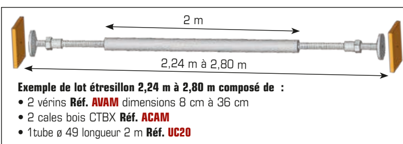
Amarrage en fenêtre avec : lot étréssillon + colliers à clavettes ou raccords à boulons + tubes + cales bois.
