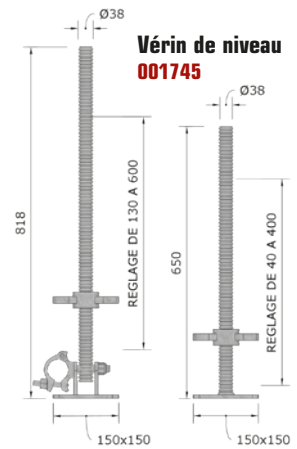
Vérin de niveau articulé 001744
