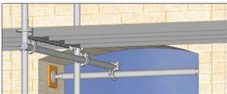
Amarrage en fenêtre avec : lot étréssillon + colliers à clavettes ou raccords à boulons + tubes + cales bois.
