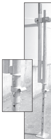
Pour rattapage de dénivellation : Platine réglable ( r é f . 0 3 4 5 ) (réglage de 27cm à 45cm)
