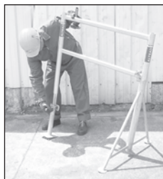
Montage d'un tréteau Dauphiné dédoublé (réf. 1924). Hauteur tréteau : 1.15m
