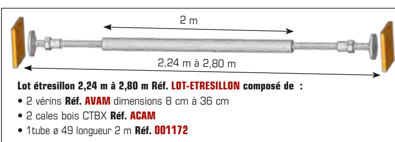
Amarrage en fenêtre avec : lot étréssillon + colliers à clavettes ou raccords à boulons + tubes + cales bois.
