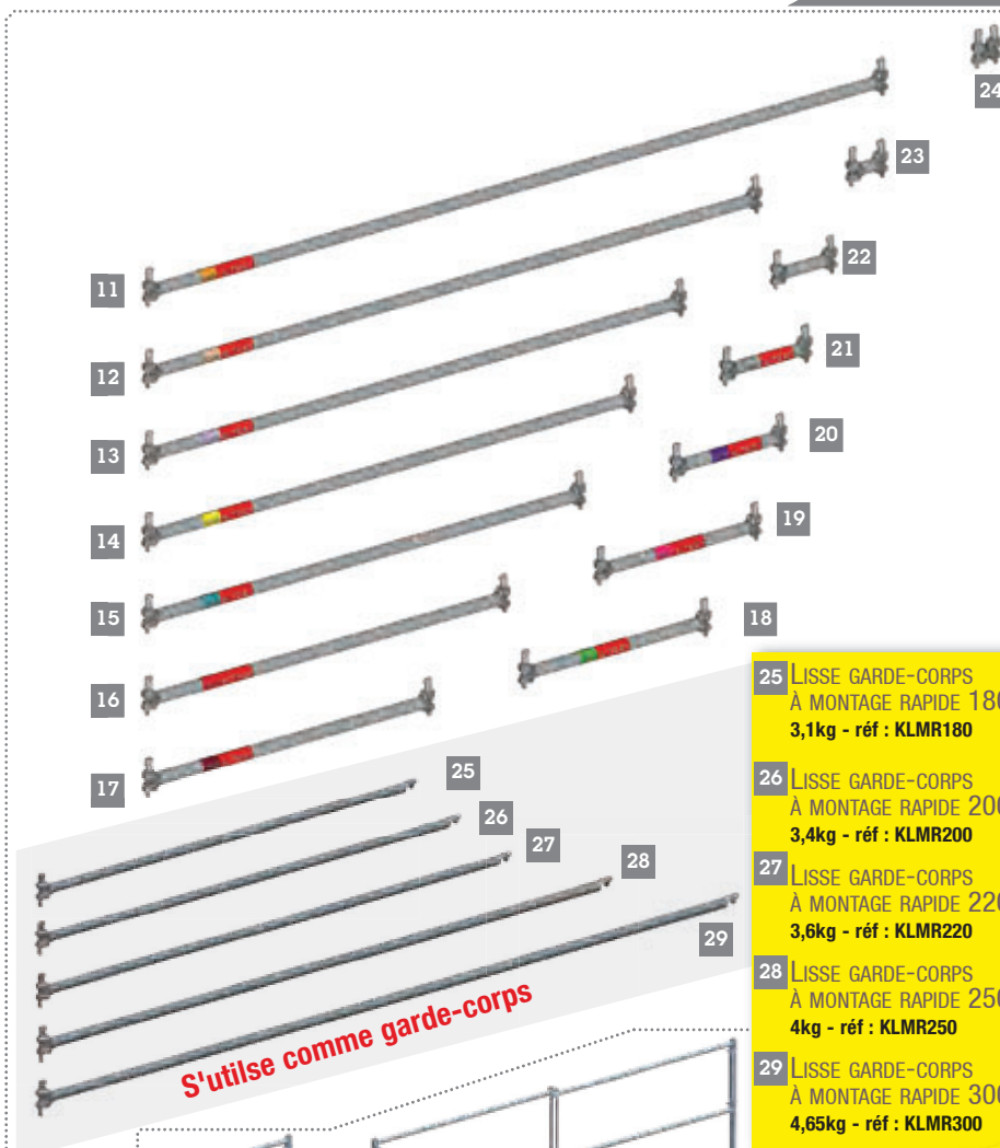
GARDE-CORPS PROVISOIRE 1500 à 3000 mm - 23,6kg - réf : 001788
